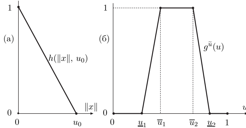
Рис. 23. Графики функций: (а) h(\|x\|, u_0) , \|x\| \in \mathbb{R}_+ = [0, +\infty) , u_0 \in U = \mathbb{R}_+ фиксировано, h(0, u) = 1 , u \in \mathbb{R}_+ ; (б) g^{\tilde{u}}(u) , u \in \mathbb{R}_+ , g^{\tilde{u}}(u) = 1 , если \bar{u}_1 \leq u \leq \bar{u}_2 , g^{\tilde{u}}(u) = 0 , если 0 \leq u \leq \underline{u}_1 или u \geq \underline{u}_2 .
