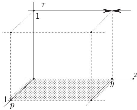
Рис. 18. График функции \tau_x^{X \setminus \tilde{A}_{(y)}}(p) , x \in X , p \in [0, 1] , (3.6).
