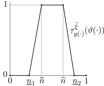
Рис. 20. График распределения \tau_{y(n)}^{\tilde{\xi}}(\vartheta(n)) , n \in [0, 1] .
