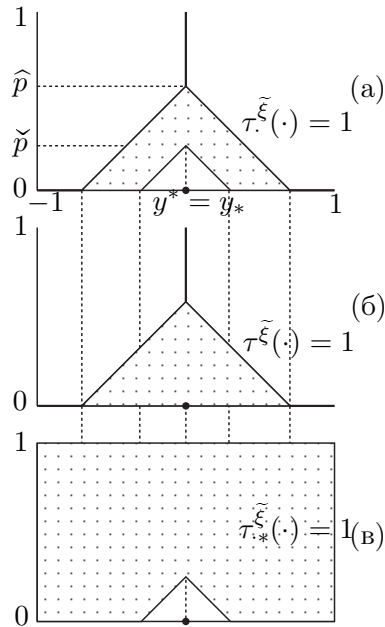
Рис. 14. Распределение \tau_{\tilde{x}}^{\tilde{\xi}}(p) , (x, p) \in [-1, 1] \times [0, 1] равно единице всюду в заштрихованной области, нулю — в незаштрихованной, (а), аналогично представлены \tau_{\tilde{x}^*}^{\tilde{\xi}}(p) , (x, p) \in [-1, 1] \times [0, 1] , (б), и \tau_{\tilde{x}^*}^{\tilde{\xi}}(p) , (x, p) \in [-1, 1] \times [0, 1] , (в); y^* = y_* — оптимальная оценка \xi , см. рис. 15.
