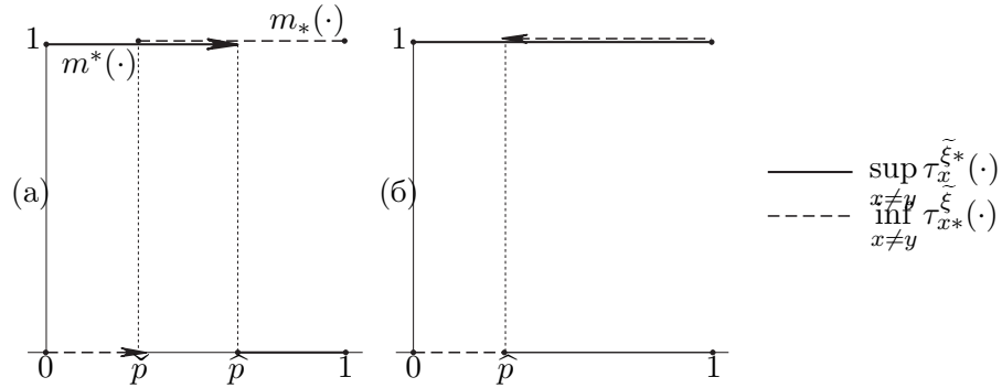
Рис. 15. Графики функций m^*(p) = \sup_{x \neq y^*} \tau_x^{\tilde{\xi}^*}(p) , p \in [0, 1] , (—), и m_*(p) = \inf_{x \neq y^*} \tau_{x^*}^{\tilde{\xi}}(p) , p \in [0, 1] , (---), y^* = y_* , (а); графики функций \sup_{x \neq y} \tau_x^{\tilde{\xi}^*}(p) , p \in [0, 1] , и \inf_{x \neq y} \tau_{x^*}^{\tilde{\xi}}(p) , p \in [0, 1] , при y \neq y^* = y_* , (б), см. рис. 14. Для наилучшей оценки y^* = y_* НН элемента \tilde{\xi} вполне правдоподобны лишь значения возможности p \in [\check{p}, \hat{p}] ошибки оценивания. Для любой другой оценки y вполне правдоподобны возможности p \in (\check{p}, 1] ошибки, в частности, вполне правдоподобна возможность p = 1 .
