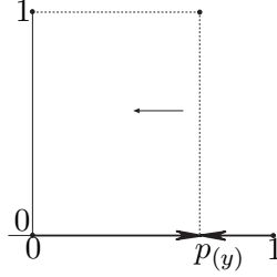
Рис. 10. График функции \text{Pl}^{(y)}(p) , p \in [0, 1] , (2.3). Стрелками \rightarrow\leftarrow выделено единственное значение p_{(y)} = P(\xi \in A_{(y)}) возможности ошибки, правдоподобие которого равно единице, правдоподобие любого другого значения возможности ошибки равно нулю. Стрелка \leftarrow указывает направление движения значения p_{(y)} при минимизации правдоподобия большой и максимизации правдоподобия малой возможности ошибки, y \in Y .
