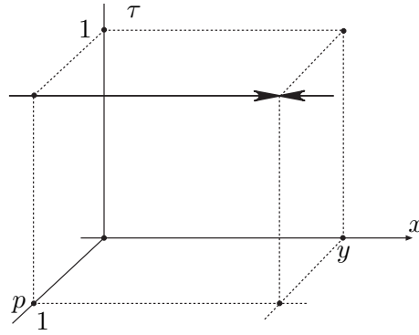
Рис. 12. График функции \tau_x^{\tilde{A}(y)}(p) , x \in X , p \in [0, 1] .
