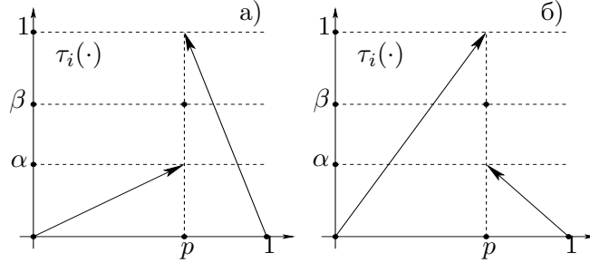
Рис. 6. Графики функций \tau_i(\cdot) , i = 1, 2, \dots
