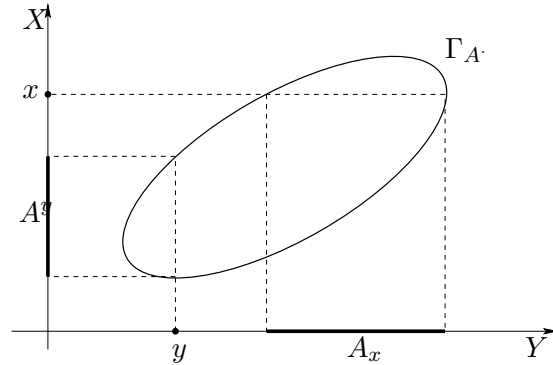
Рис. 7. График \Gamma_A отображения A: Y \rightarrow \mathcal{P}(X) ; множества A^y \subset X , A_x \subset Y
