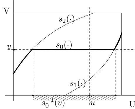
Рис. 5. Жирной линией выделена функция s_0(\cdot) , на которой достигается \sup в (4.11), равный g^{\tilde{v}}(v) = \sup_{u \in s_0^{-1}(v)} g^{\tilde{u}}(u)
