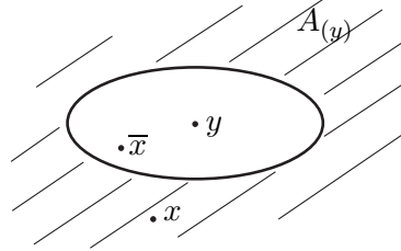
Рис. 8. Элемент x \in X покрыт, элемент \bar{x} \in X — не покрыт множеством A_{(y)} , которое является значением НН множества \tilde{A}_{(y)} при y \in Y , (см. ч. I).
