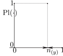
Рис. 16. Стрелками \rightarrow\leftarrow отмечено единственное значение n_{(y)} = N(\xi \in A_{(y)}) необходимости ошибки оценивания ОН элемента \tilde{\xi} значением y \in Y , правдоподобие которого равно единице, другие значения необходимости ошибки — неправдоподобны.
