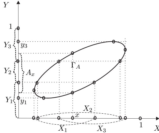
Рис. 3. График нечеткого множества, индикаторная функция которого не определена для любого x \in X_1 \cup X_2 \cup X_3 , множества Y_1, Y_2, Y_3 образуют разбиение Y = Y_1 \cup Y_2 \cup Y_3 = [0, 1] , X \in [0, 1] .
