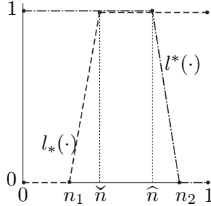
Рис. 19. Графики функций l_*(n) , n \in [0, 1] , и l^*(n) , n \in [0, 1] .
