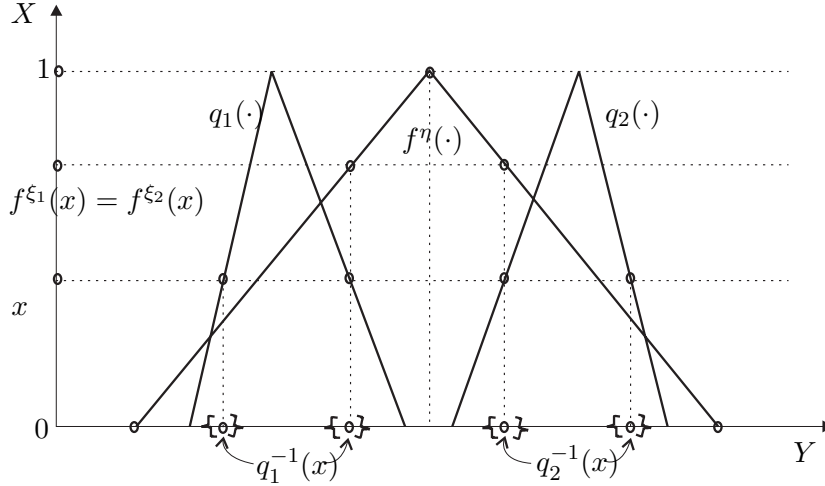
Рис. 1. В силу симметрии функций f^\eta(\cdot) , q_1(\cdot) и q_2(\cdot) , показанной на рисунке, f^{\xi_1}(x) = f^{\xi_2}(x) , x \in X , в то время как q_1(y) \neq q_1(y) , y \in Y .
