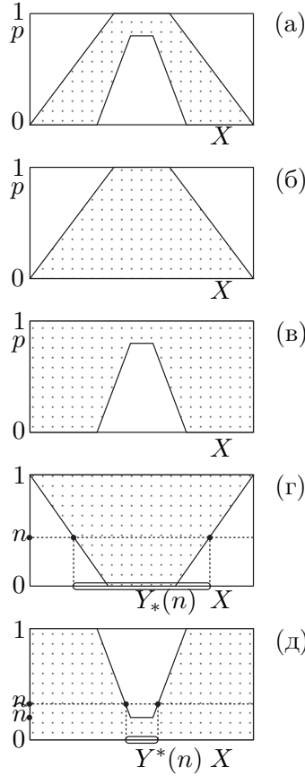
Рис. 21. (а) \tau_x^{\tilde{\xi}}(p) = 1, (x, p) \in (\text{заштрихованная область}) \subset X \times [0, 1]; \tau_x^{\tilde{\xi}}(p) = 0, (x, p) \in (X \times [0, 1]) \setminus (\text{заштрихованная область}). (б) \tau_x^{\xi^*}(p) = 1, (x, p) \in (\text{заштрихованная область}) \subset X \times [0, 1]; \tau_x^{\xi^*}(p) = 0, (x, p) \in (X \times [0, 1]) \setminus (\text{заштрихованная область}). (в) \tau_{x^*}^{\tilde{\xi}}(p) = 1, (x, p) \in (\text{за-} \text{штрихованная область}) \subset X \times [0, 1]; \tau_{x^*}^{\xi}(p) = 0, (x, p) \in (X \times [0, 1]) \setminus (\text{за-} \text{штрихованная область}). (г) \tau_x^{\tilde{\xi}^*}(\vartheta(n)) = 1, (x, n) \in (\text{заштрихованная} \text{область}) \subset X \times [0, 1]; \tau_x^{\tilde{\xi}^*}(\vartheta(n)) = 0, (x, n) \in (X \times [0, 1]) \setminus (\text{заштрихо-} \text{ванная область}). (д) \tau_{x^*}^{\xi}(\vartheta(n)) = 1, (x, n) \in (\text{заштрихованная об-} \text{ласть}) \subset X \times [0, 1]; \tau_{x^*}^{\xi}(\vartheta(n)) = 0, (x, n) \in (X \times [0, 1]) \setminus (\text{заштрихованная} \text{область}). Y^*(n) \subset Y_*(n), n > \hat{n}; Y = X, Y^*(n) \supset Y_*(n), n < \hat{n}.
