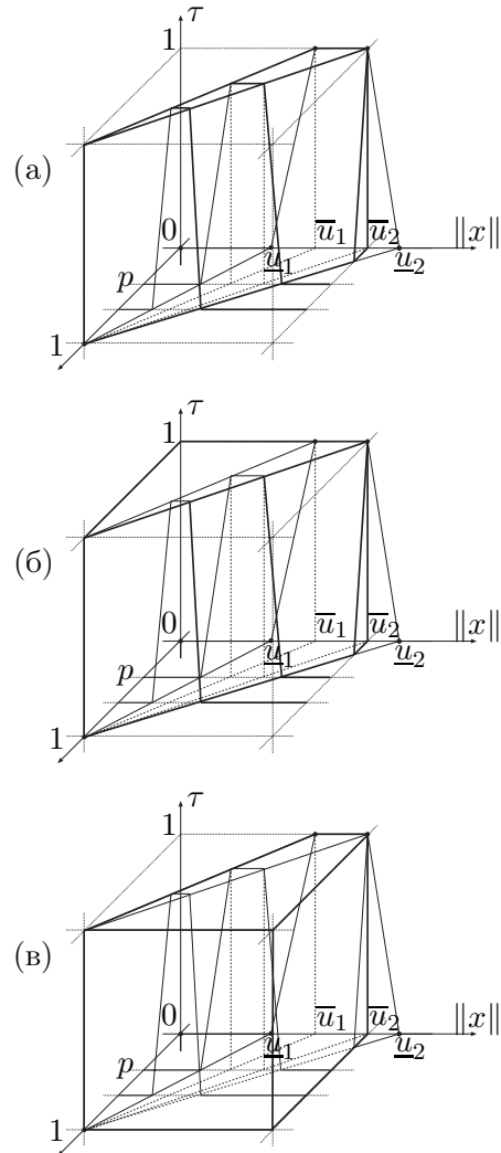
Рис. 24. (а) График функции (поверхность) \tau_x^{\bar{\nu}}(p) , x \in X , p \in [0, 1] . Приведена зависимость от \|x\| \in [0, \infty) , \|x\| \in [0, \bar{u}_2] и p \in [0, 1] . (б) График функции (поверхность) \tau_x^{\bar{\nu}^*}(p) , x \in X , p \in [0, 1] . Показаны зависимости от \|x\| \in [0, \infty) , \|x\| \in [0, \bar{u}_2] и p \in [0, 1] . (в) График функции (поверхность) \tau_{x^*}^{\bar{\nu}}(p) , x \in X , p \in [0, 1] . Показаны зависимости от \|x\| \in [0, \infty) , \|x\| \in [0, \bar{u}_2] и p \in [0, 1] .
