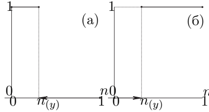
Рис. 17. Графики функций \text{Pr}(N(\tilde{\xi} \in \tilde{A}_{(y)}) \geq n) , n \in [0, 1] , (а), и \text{Pr}(N(\tilde{\xi} \in \tilde{A}_{(y)}) \leq n) , n \in [0, 1] , (б). При любом y \in Y_0 n_{(y)} = 0 .
