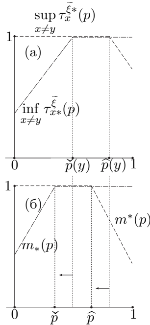
Рис. 13. Графики функций \inf_{x \neq y} \tau_{x^*}^{\tilde{\xi}}(p) , \sup_{x \neq y} \tau_x^{\tilde{\xi}^*}(p) , m_*(p) и m^*(p) , p \in [0, 1] . Стрелки \leftarrow указывают смещения \check{p}(y) и \hat{p}(y) к значениям \check{p} и \hat{p} соответственно, определяемым при решении задачи (2.13). Значения возможности p \in (\check{p}, \hat{p}) ошибки вполне правдоподобны; значения, меньшие \check{p} и бóльшие \hat{p} — сомнительны.
