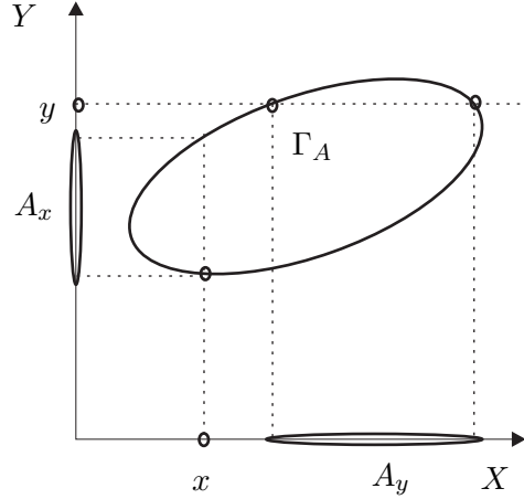
Рис. 2. Отображение A : Y \rightarrow \mathcal{P}(X) , его график \Gamma_A \subset Y \times X и обратное к A отображение A : X \rightarrow \mathcal{P}(Y) .
