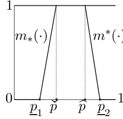
Рис. 9. Графики функций m^*(\cdot) и m_*(\cdot)
