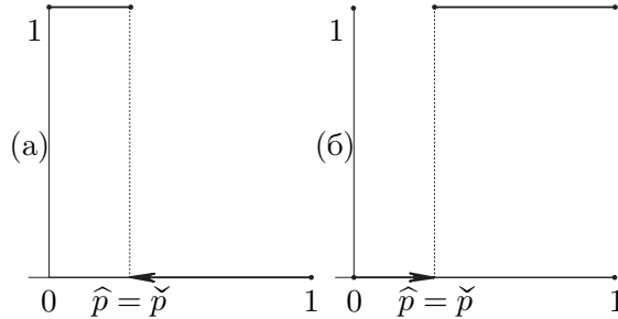
Рис. 11. Графики \text{Pl}(P(\tilde{\xi} \in \tilde{A}_{(y)}) \geq p) , p \in [0, 1] , (а), и \text{Pl}(P(\tilde{\xi} \in \tilde{A}_{(y)}) \leq p) , p \in [0, 1] , (б), при любом значении y \in \{y \in Y, P(\xi \in A_{(y)}) = \min_{\bar{y} \in Y} \sup_{x \in X} \min(f^{\xi}(x), f^{A(\bar{y})}(x))\} = Y_* = Y^* , минимизирующем возможности ошибки при оценивании нечеткого элемента \xi значением y \in Y .
