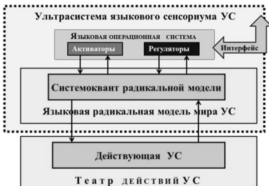
Рис. 1. Языковой сенсориум УС как ультрасистема интеллектуального планирования и ситуационного управления поведением УС
