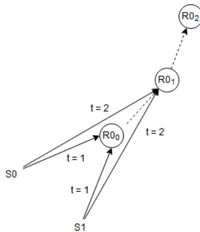
Рис. 1. Графическое представление процесса обучения нейрона
