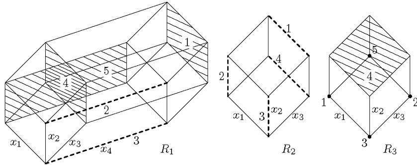
Рис. 1. Функции граневого разбиения R_1 , R_2 и R_3 .
