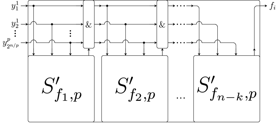
Рис. 3: Схема G_{f,p} , реализующая функцию f'' .
