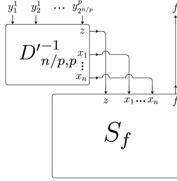
Рис. 2: Реализация схемы S'_{f,p} .
