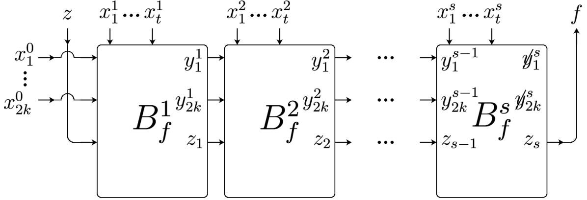
Рис. 10: Схема SL_f^s , реализующая функцию \tilde{f}' .
