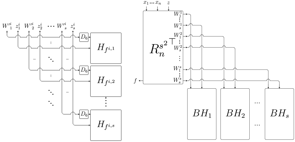
(a) Блок BH^i , реализующий функции f^{i,1}, \dots, f^{i,s} . Здесь D_6 := D'_{k/2,6}^{-1 \top} .
