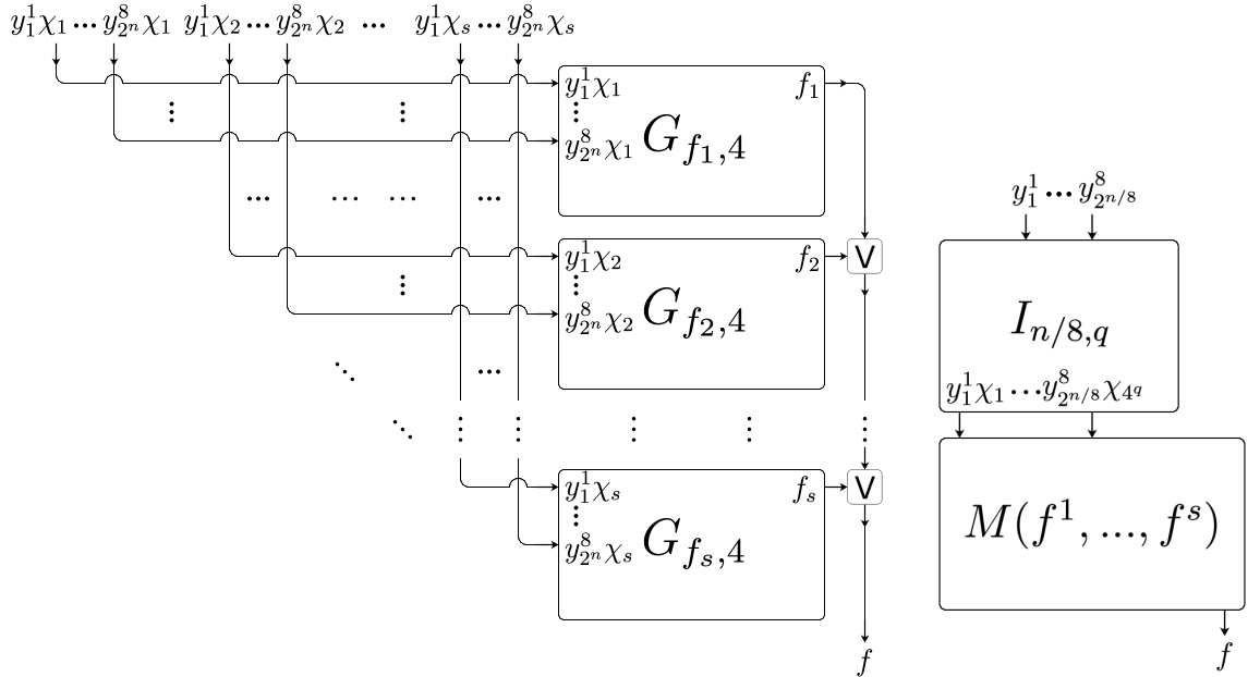
(a) Блок M(f^1, \dots, f^s) , реализующий функции \bigvee_{j=1}^s \chi_j f_8^{j''}(\vec{y}) .
