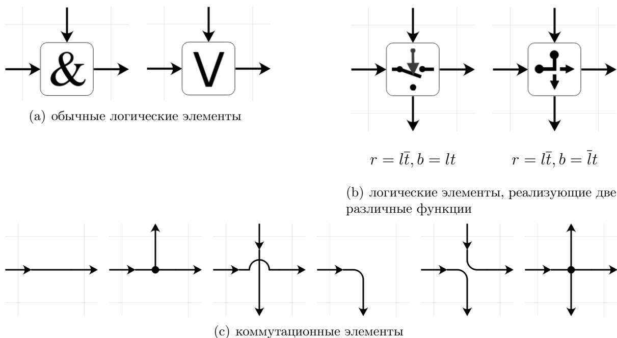
Рис. 1: Примеры клеточных элементов.
