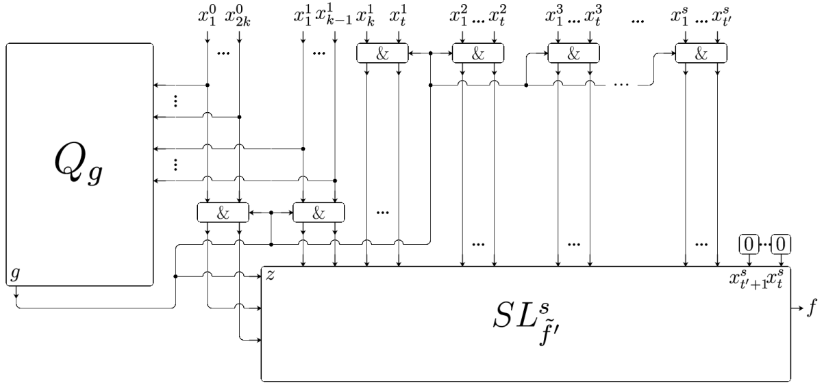
Рис. 11: Схема SF_f^h , реализующая функцию f' .
