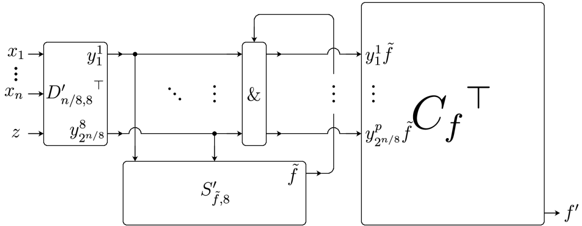
Рис. 6: Блок H_f , реализующий функцию f' .
