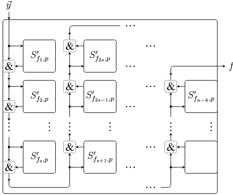
Рис. 4: Квадратная схема \tilde{G}_{f,p} , реализующая f''_p .
