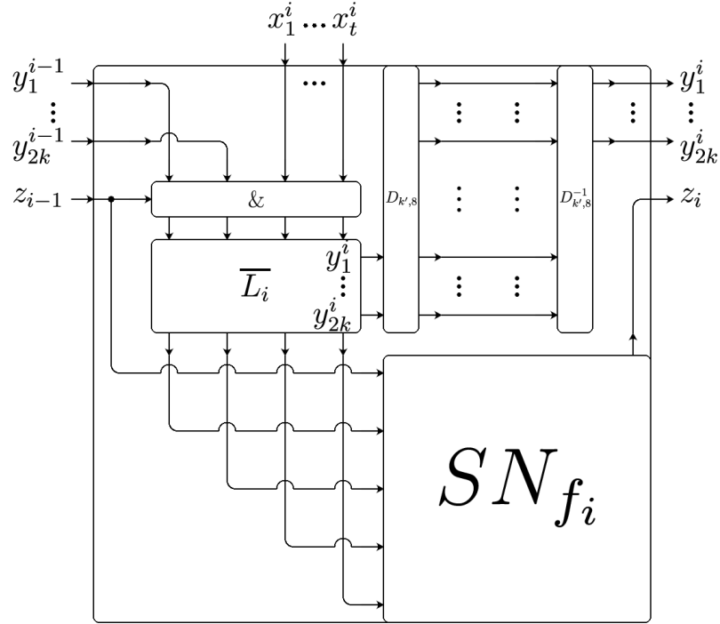
Рис. 9: Блок B_f^i , реализующий функции f^i и l_i .
