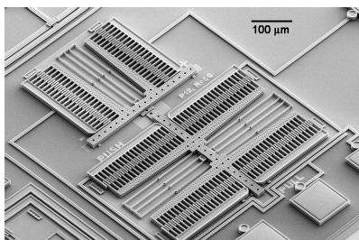
Рис. 3. Микроснимок компоненты МЭМС для измерения ускорения
