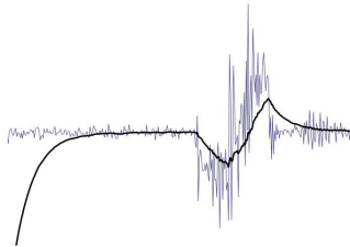
Рис. 2. Скользящее среднее с параметром \alpha = 0.95
